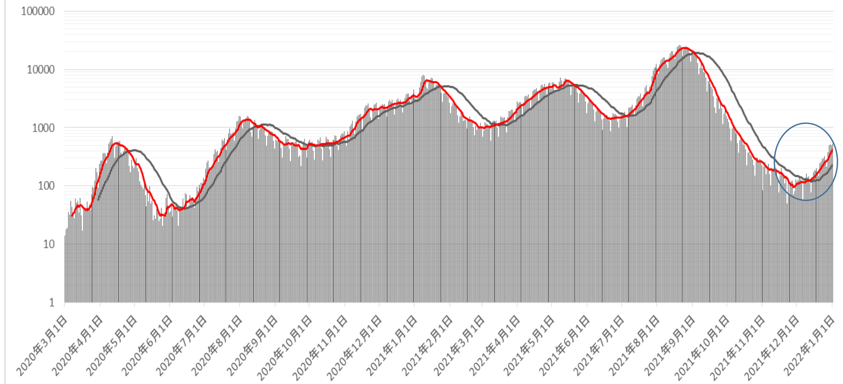
図1 縦軸を対数目盛にした7日移動平均及び30日移動平均の近似曲線の推移
