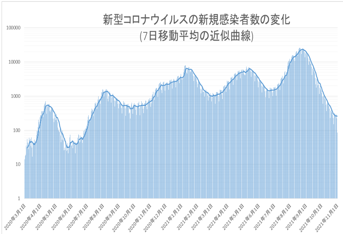
図1 縦軸を対数目盛にした7日移動平均の近似曲線の推移
